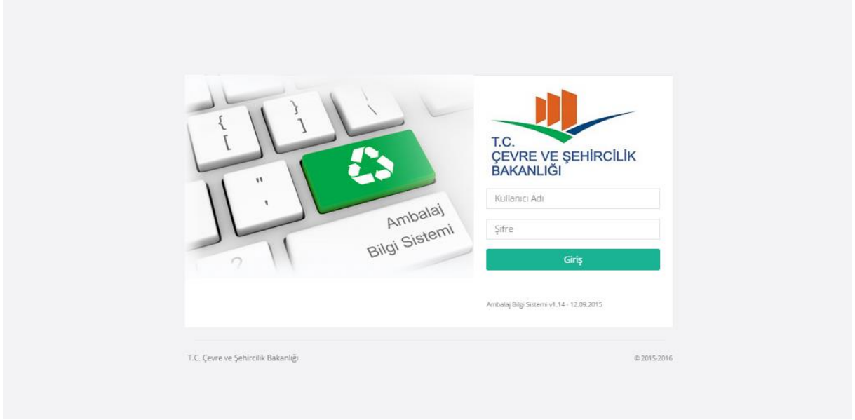
ŞEKİL 1-SİSTEM GİRİŞ SAYFASI
